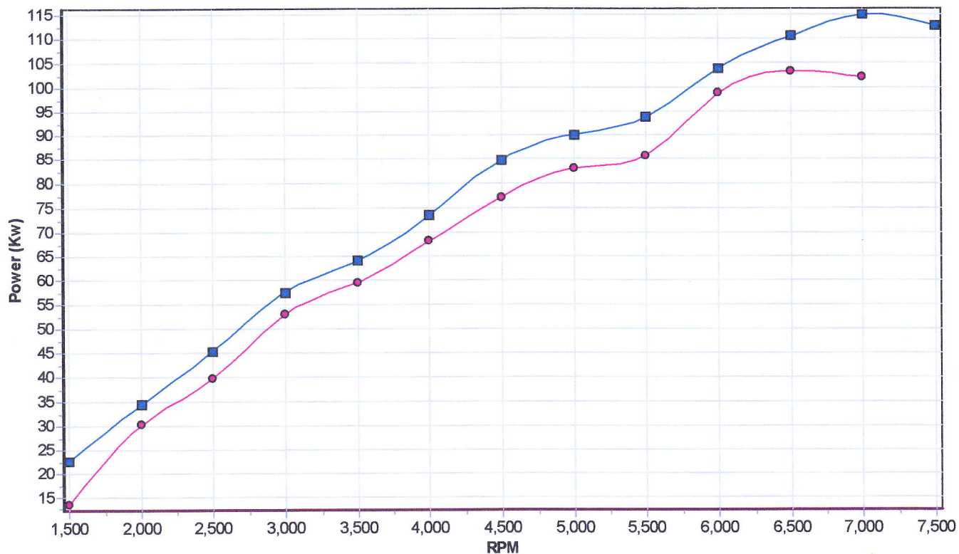
Power (Kw)
