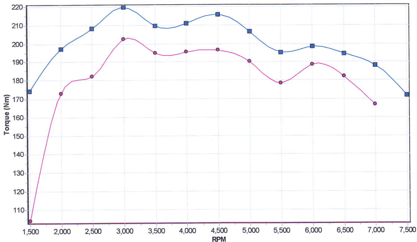
Torque (Nm)
